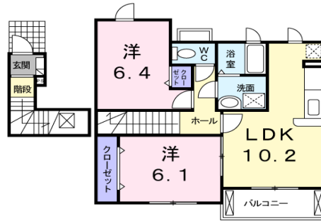
【間取り図】
